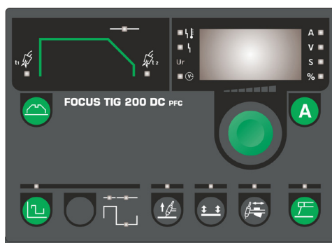
Betjeningspanel til Focus TIG 200 DC HP PFC
