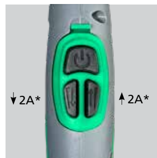
Up/Down modul med 3-knap-tast til justering af svejsestrøm. Svejsestrømmen forøges/reduceres med 2 amperet. Langt tryk for konstant forøgelse/reducering. 80300064
