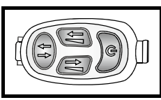
Up/Down modul med 4-knap-tast til justering af svejsestrøm inkl. TIG-A Tack funktion Up/Down module with 4-function key for adjustment of welding current incl. TIG-A-Tack function 80300063 (released after Oct. 2012)
