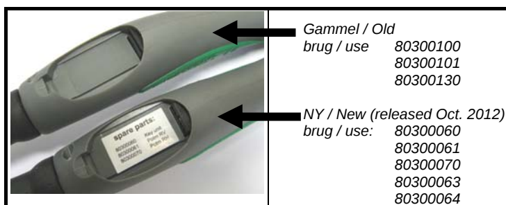
Up/Down modul med 4-knap-tast til justering af svejsestrøm inkl. TIG-A Tack funktion Up/Down module with 4-function key for adjustment of welding current incl. TIG-A-Tack function 80300063 (released after Oct. 2012)
